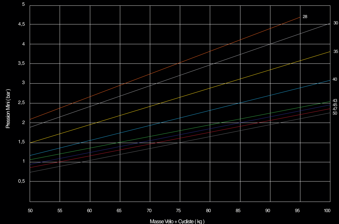
PRESSION MINIMALE JANTE EN FONCTION DE LA SECTION DU PNEUMATIQUE ET LA MASSE DU CYCLISTE
