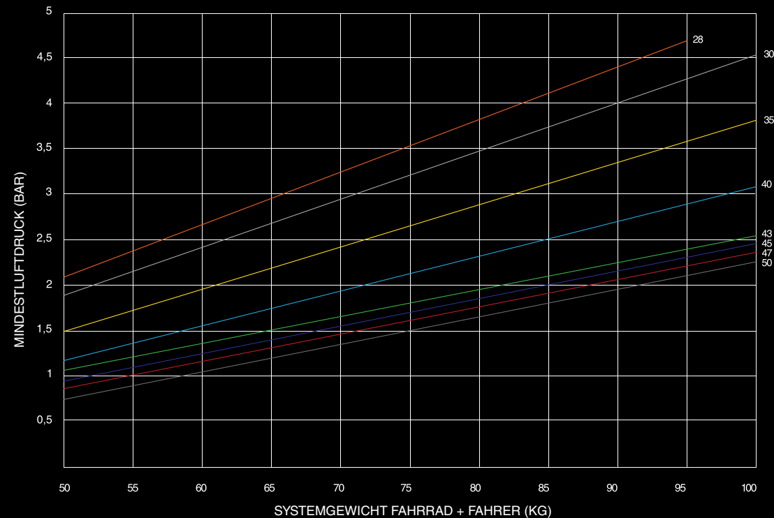
MINDESTREIFENDRUCK ENTSPRECHEND DER REIFENBREITE UND DEM GEWICHT DES FAHRRADFAHRERS
